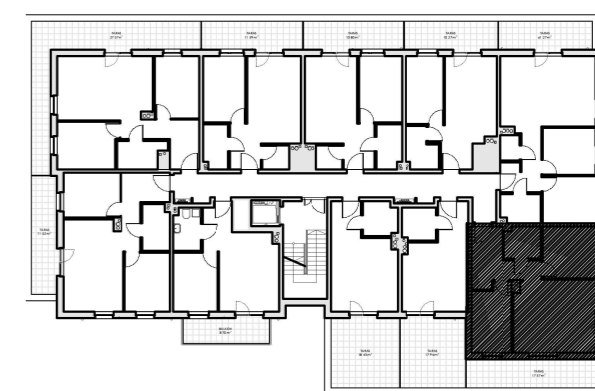
RZUT KONDYGNACJI Z ZAZNACZENIEM LOKALU MIESZKALNEGO
