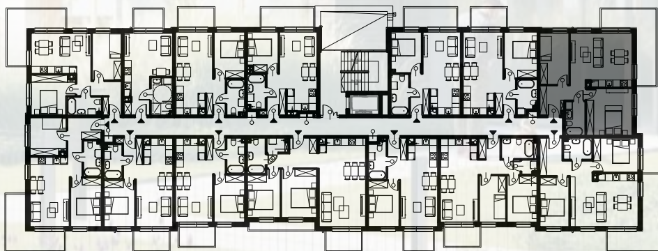
SCHEMAT KONDYGNACJI
