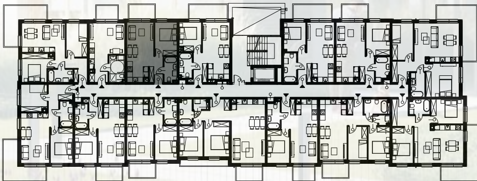
SCHEMAT KONDYGNACJI
